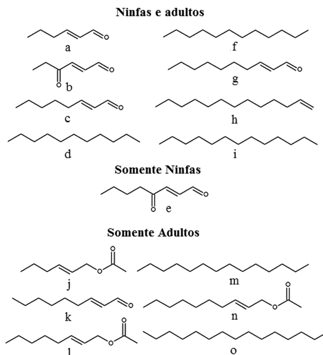
Figura 3. Estruturas químicas dos compostos presentes nas DAGs das ninfas e na MTG dos adultos das espécies L. deducta e P. stictica . a: (E)-2-hexenal, b: (E)-4-oxo-2-hexenal, c: (E)-2-octenal, d: undecano, e: (E)-4-oxo-2-octenal, f: dodecano, g: (E)-2-decenal, h: 1-trideceno, i: tridecano, j: acetato de (E)-2-hexenila, k: (E)-2-nonenal, l: acetato de (E)-2-octenila, m: tetradecano, n: acetato de (E)-2-decenila, o: pentadecano
